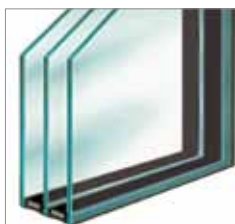
Wärmeschutzglas, 3-fach Therm Ultra 0.7 WE Glasaufbau 4-12-4-12-4 mm U_g: 0,7 \text{ W/m}^2 \text{ K} R_w: 35 \text{ dB}
